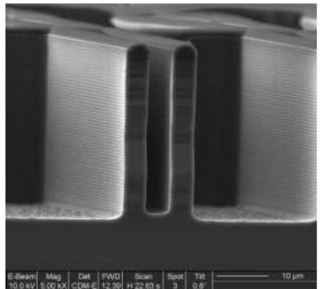
トレンチエッチングシリコン
